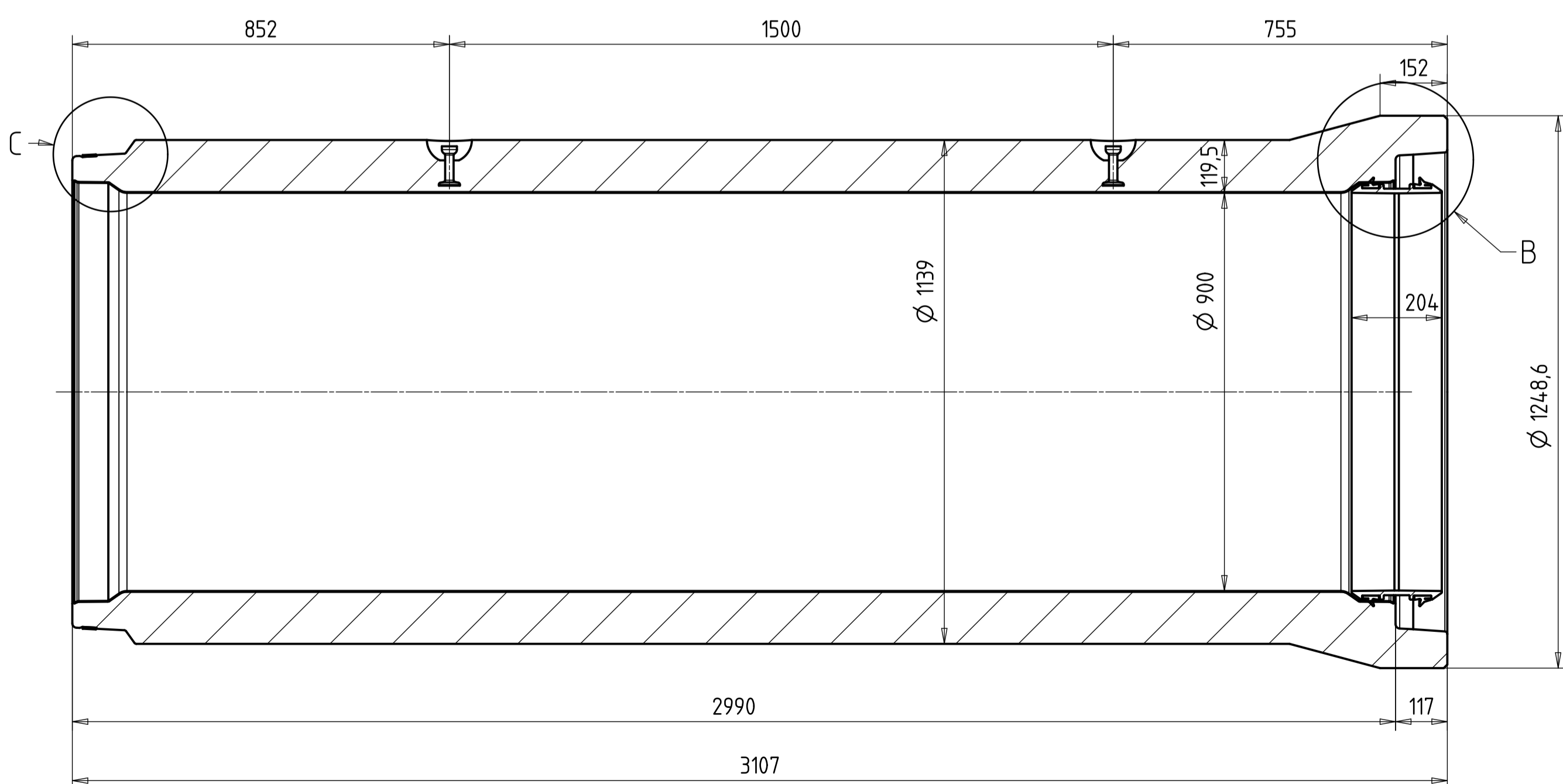
SCHNITT A-A
